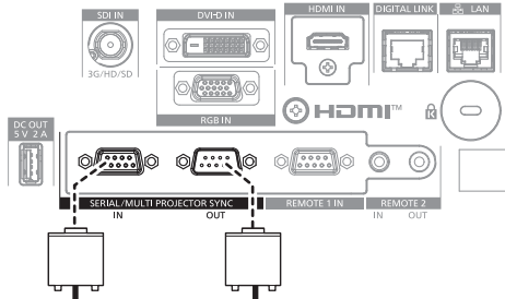
Anschlüsse des vierten Projektors
