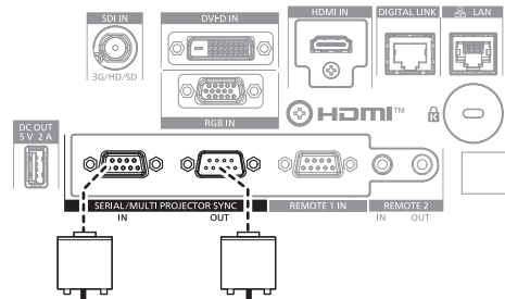
Anschlüsse des zweiten Projektors
