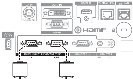
Anschlüsse des ersten Projektors
