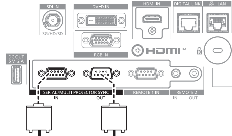
Anschlüsse des dritten Projektors
